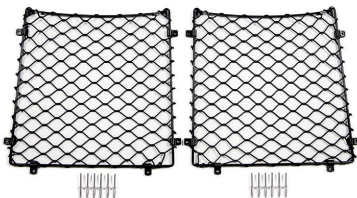
Plasă transport, ușa din spate - 7TG017230
